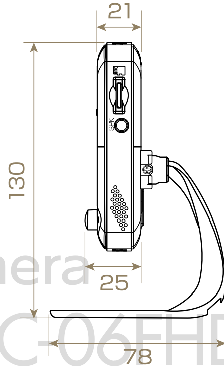
【側面】
