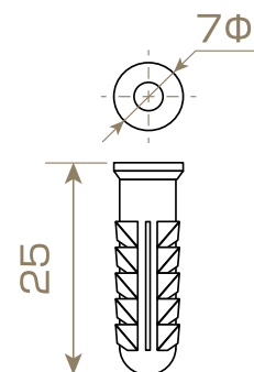
【アンカー】
