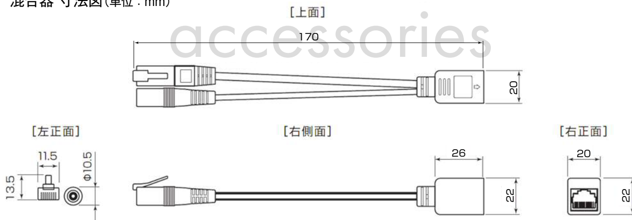
混合器 寸法図 (単位 : mm)
