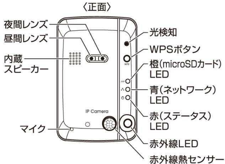
図 3-1:正面各部
