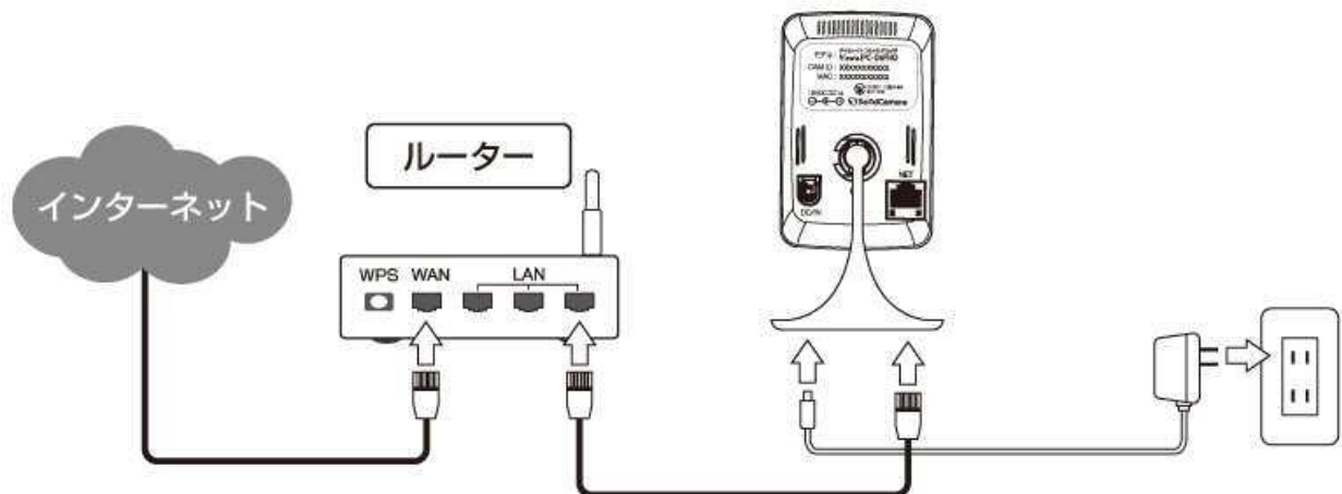
図 3-4:IPC-06FHD-T 接続図
