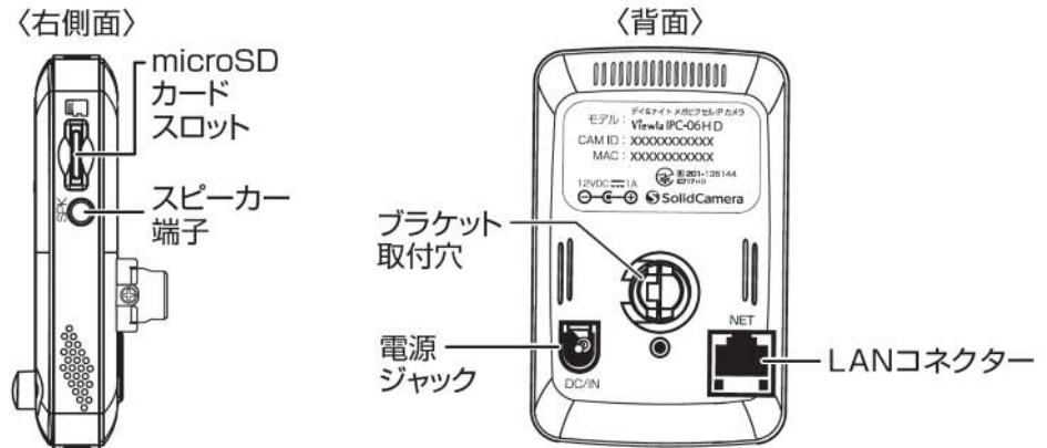
図 3-2: 右側面・背面各部
