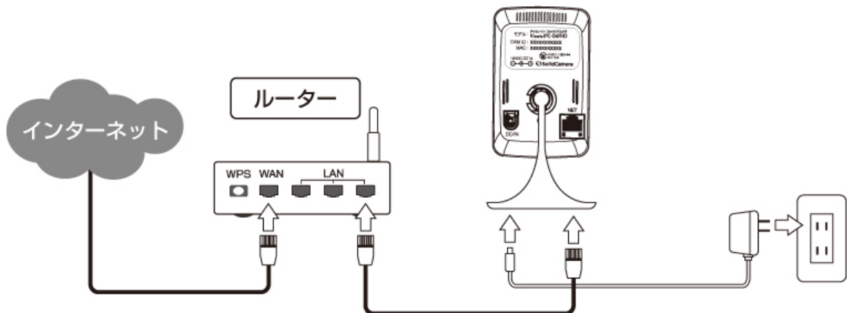
図 3-4:IPC-06FHD-T 接続図
