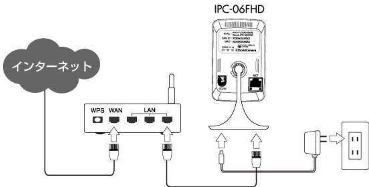
図 3-4:IPC-06FHD 接続図
