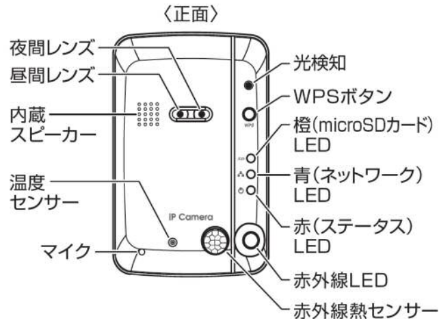
図 3-1: 正面各部
