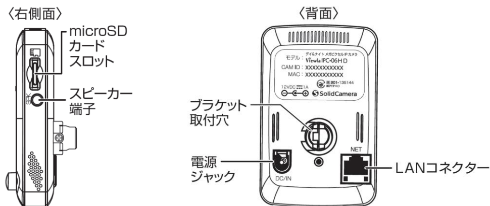
図 3-2：右側面・背面各部
