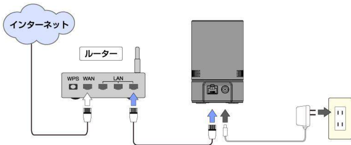
図 3-3 : IPC-08FHD 接続図
