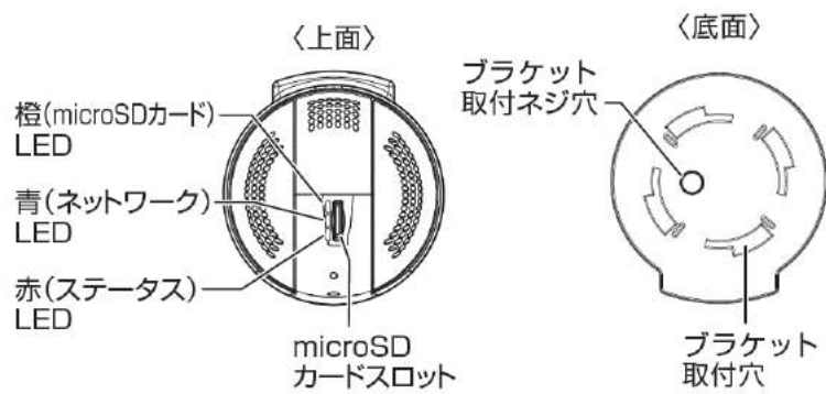
図 3-2：上面・底面各部
