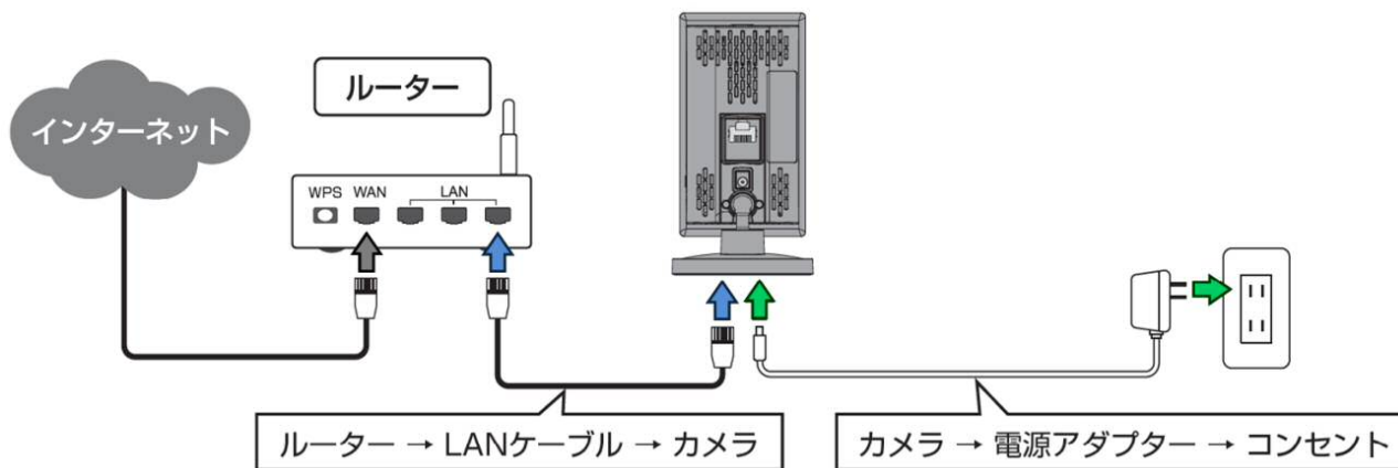
図 3-3 : IPC-09w 接続図
