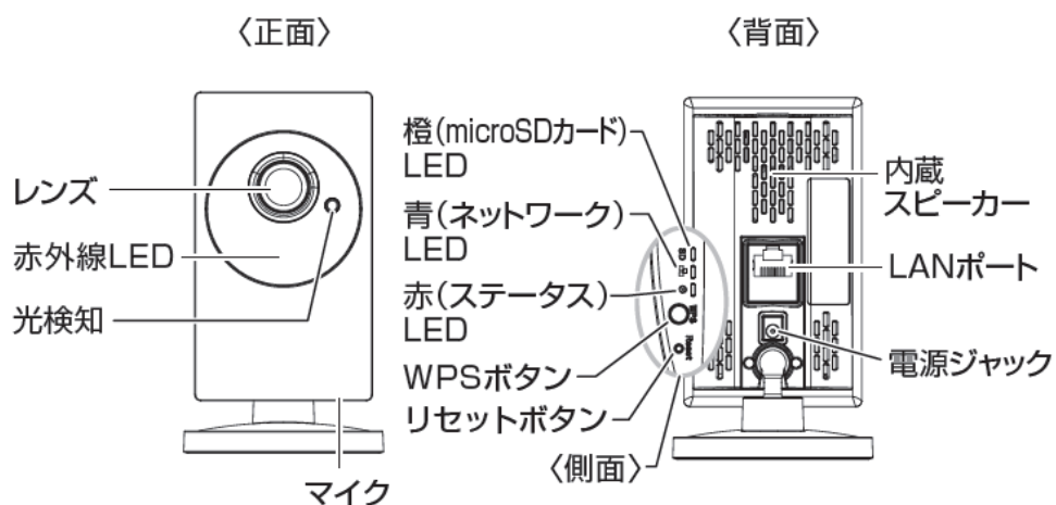
図 3-1：正面・背面各部
