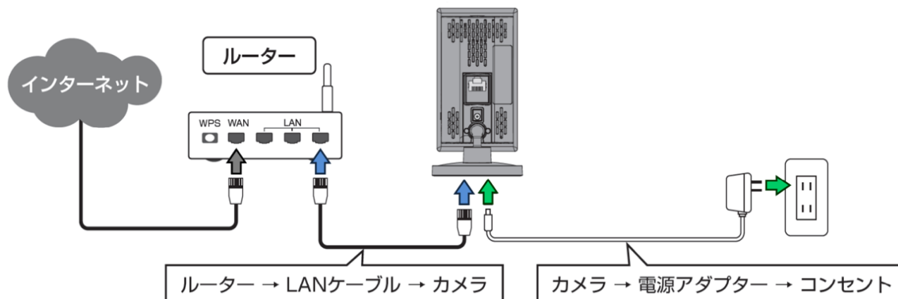
図 3-3 : IPC-09wp 接続図
