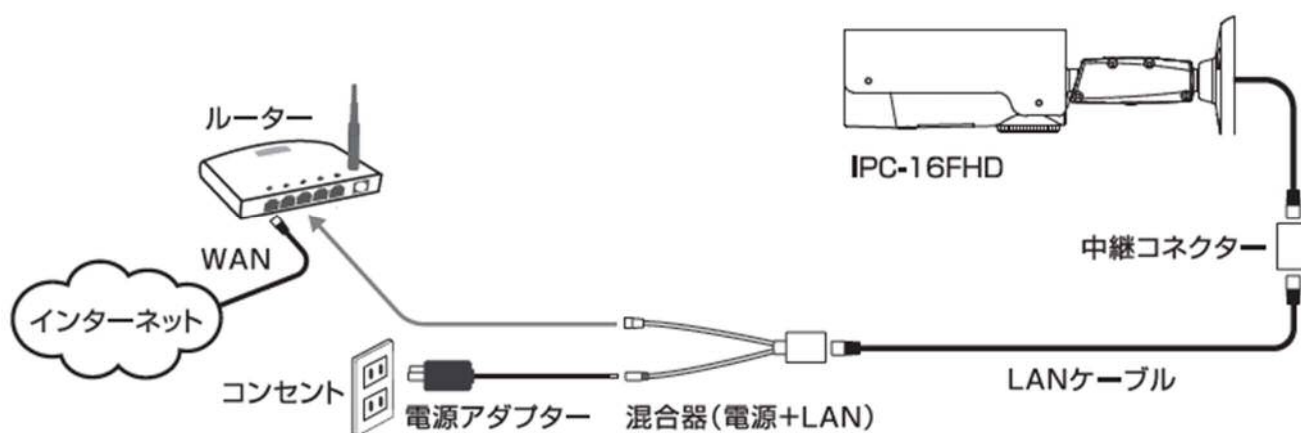
図 3-4 : IPC-16FHDp 接続図
