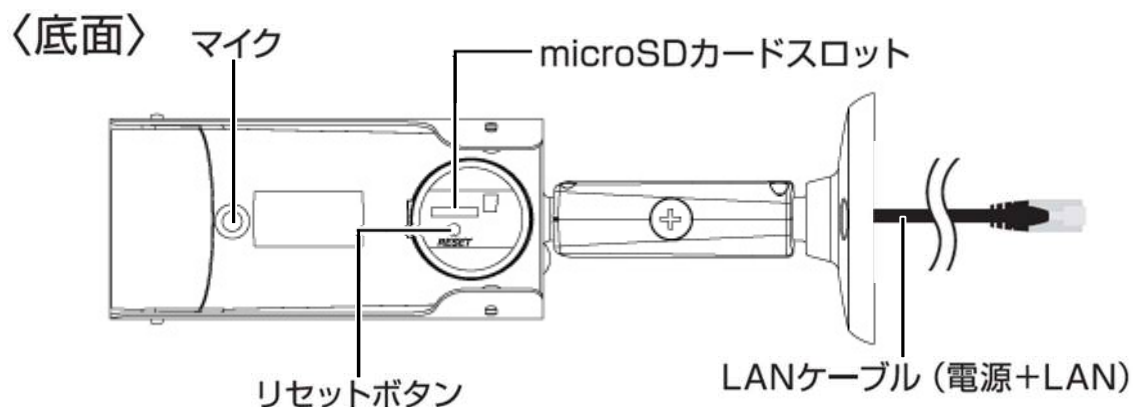
図 3-2 : 底面各部
