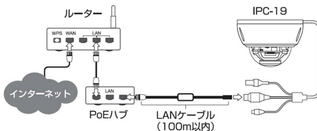
図 3-6 : IPC-19 接続図 1
