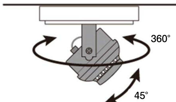
図 3-4 : レンズの可動域
