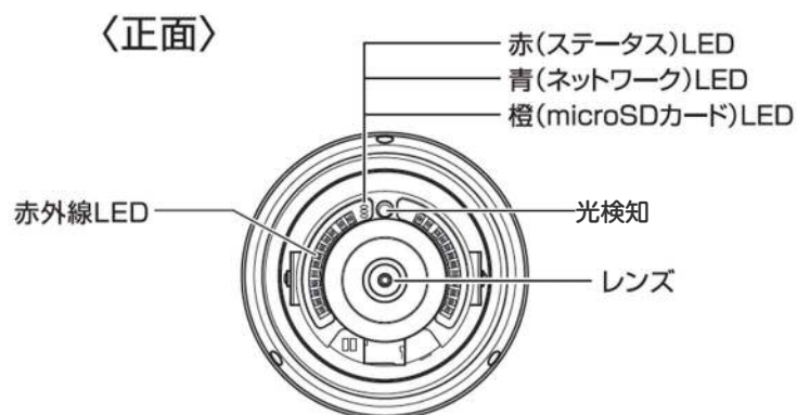
図 3-1 : 正面各部
