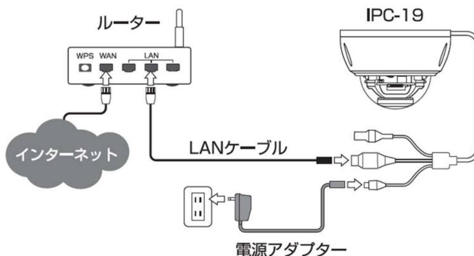
図 3-7 : IPC-19 接続図 2
