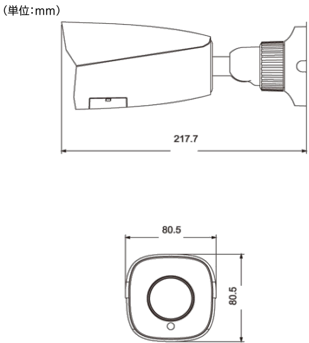
寸法図
